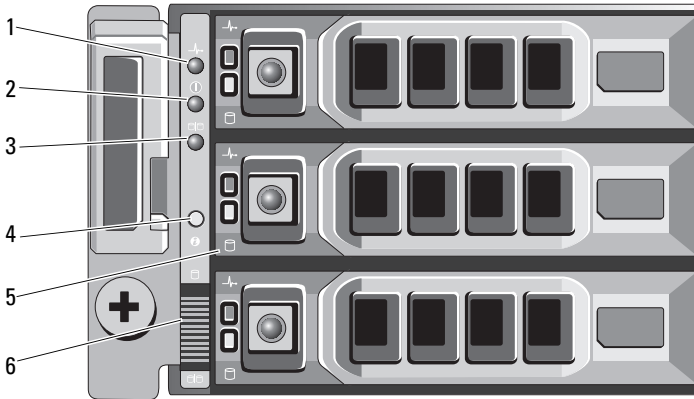
Ilustración 2-1. Indicadores y funciones del panel anterior: Dell PowerVault MD3620i
