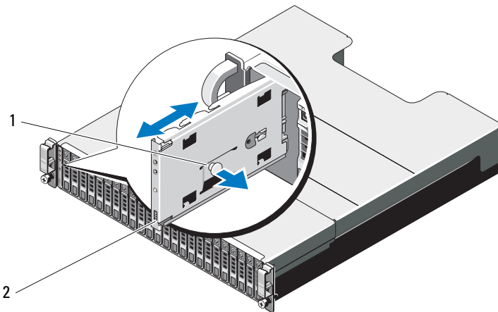
Ilustración 16-14. Extracción e instalación del panel de control de PowerVault MD3620i
