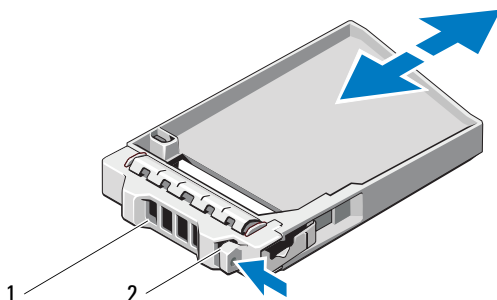
Ilustración 16-3. Extracción e instalación de una unidad de disco duro de relleno de 2,5 pulgadas (solo MD3620i)
