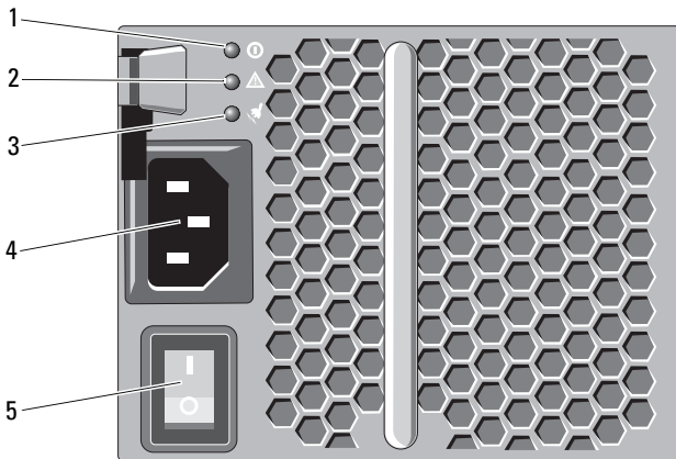
Ilustración 2-6. Funciones y códigos del indicador de alimentación
