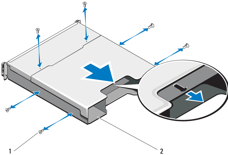
Ilustración 16-15. Extracción e instalación del alojamiento para el módulo de la controladora RAID/suministro de energía
