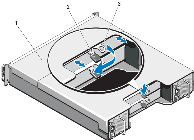
Ilustración 16-8. Extracción e instalación de un módulo de controladora RAID
