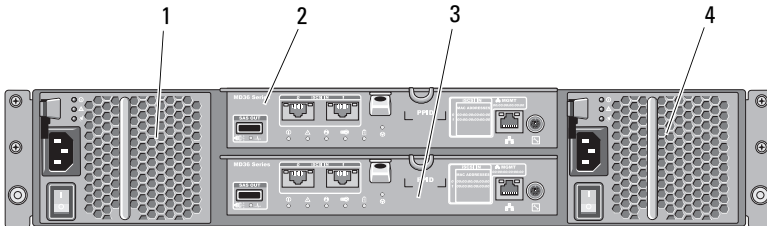
Ilustración 2-4. Indicadores y funciones del panel posterior de la matriz de almacenamiento Dell PowerVault MD3600i
