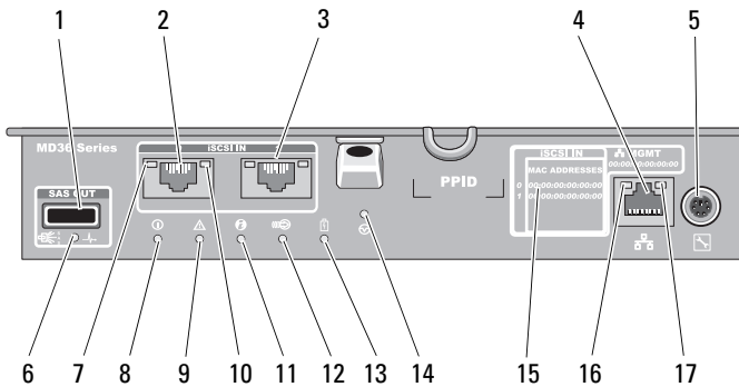
Ilustración 3-1. Módulo de la controladora RAID iSCSI serie MD3600i
