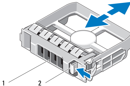
Ilustración 16-2. Extracción e instalación de una unidad de disco duro de relleno de 3,5 pulgadas (solo MD3600i)
