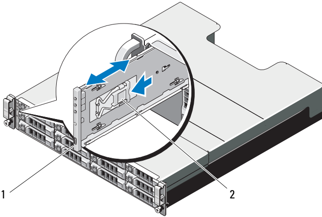
Ilustración 16-13. Extracción e instalación del panel de control de PowerVault MD3600i
