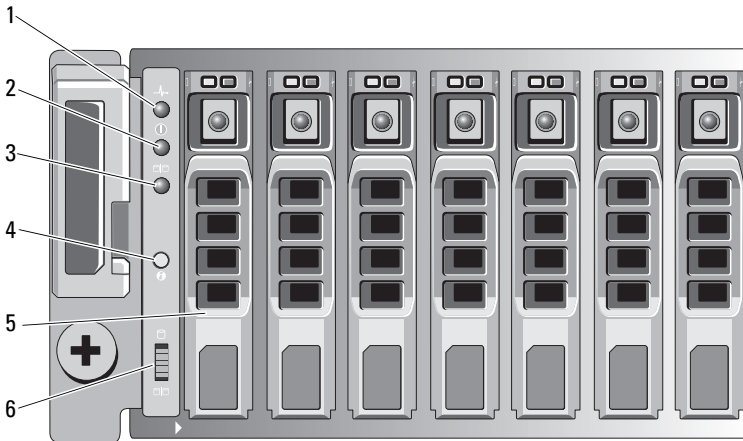
Ilustración 2-2. Indicadores y funciones del panel anterior: Dell PowerVault MD3620i
